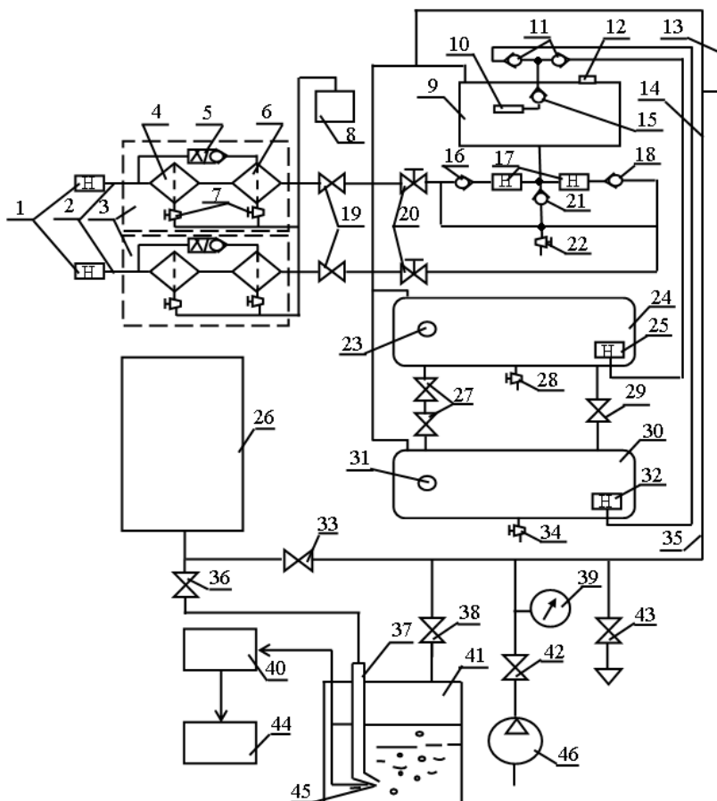
Зураг-2. Түлшний систем болон түүний битүүмжлэл шалгах төхөөрөмжийн зарчмын бүдүүвч
