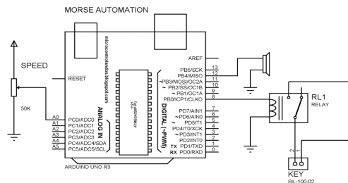
Зураг 4. Цахилгааны бүдүүвч /Protues 8.1/
