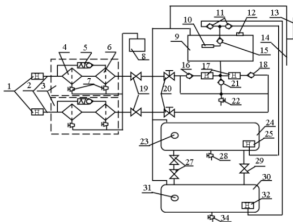
Зураг-1. Ми-8 нисдэг тэрэгний түлшний системийн зарчмын бүдүүвч
