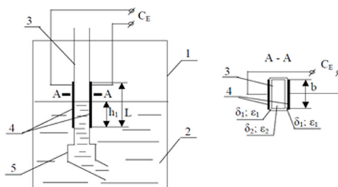
Зураг 4. Хөөс хэмжигч
