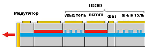
Зураг 6. Оптик радио хувиргагч /нэвтрүүлэгч/
