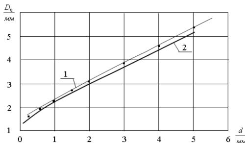
Зураг-3. 1 – туршилтын муруй, 2 – онолын муруй ( D – хөөсний диаметр, d – хөөсрүүлэх хоолойн дотоод диаметр)
