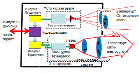
Зураг 7. Оптик радио системийн ажиллагааны зарчим
