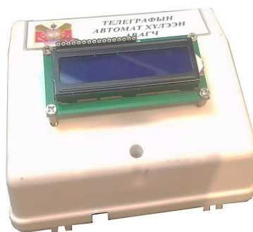
Зураг 9. Телеграфын автомат хүлээн авагч
