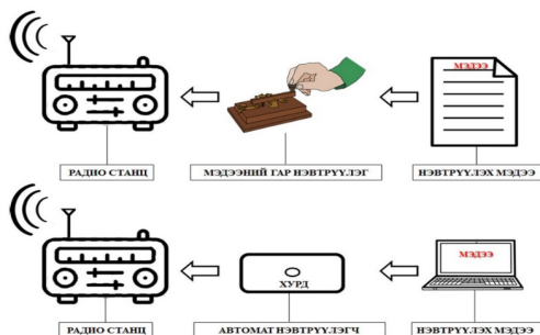
Зураг 1 Радио телеграфыг нэвтрүүлэх ажиллагаа
