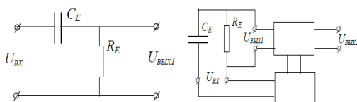
Зураг-5. Хөөс хэмжигчийн дифференциал хэлхээ
