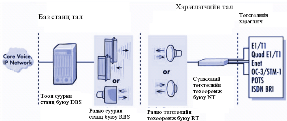
1 дүгээр зураг. LMDS системийн дамжууллын ерөнхий блок схем
