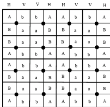
2 дугаар зураг. 2 давтамж дахин ашигласан давтамж төлөвлөлт
