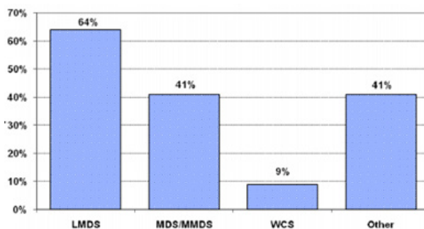
3 дугаар зураг. 2.3GHz дээш давтамж ашигладаг утасгүй холбооны системүүд
