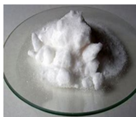
Гуравдугаар зураг. Калийн нитрат - KNO_3 65%
