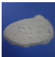
Аравдугаар зураг. KNO_3 болон C_6H_{14}O_6 .
