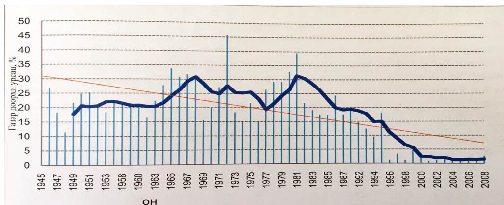
Туул голын ай сав газрын урсац газрын доорх усаар тэжээгдэх байдлын өөрчлөлтийн хөдлөлзүйн муруй
