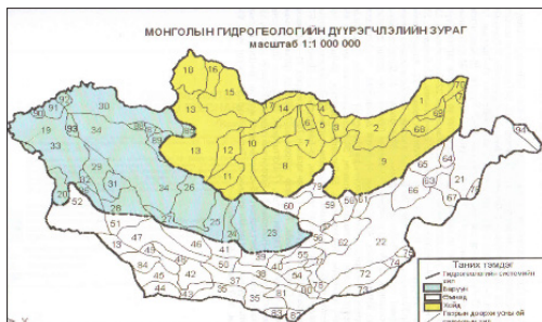
1 дүгээр зураг. Монгол орны усны 29 ай сав газар болон дүүрэгчилсэн зураглал (саарал өнгөтэй нь нөхөн сэргээгддэггүй нөөц тархсан газрууд)
