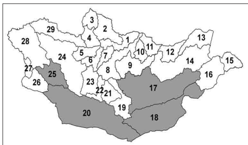
1 дүгээр зураг. Монгол орны усны 29 ай сав газар болон дүүрэгчилсэн зураглал (саарал өнгөтэй нь нөхөн сэргээгддэггүй нөөц тархсан газрууд)
